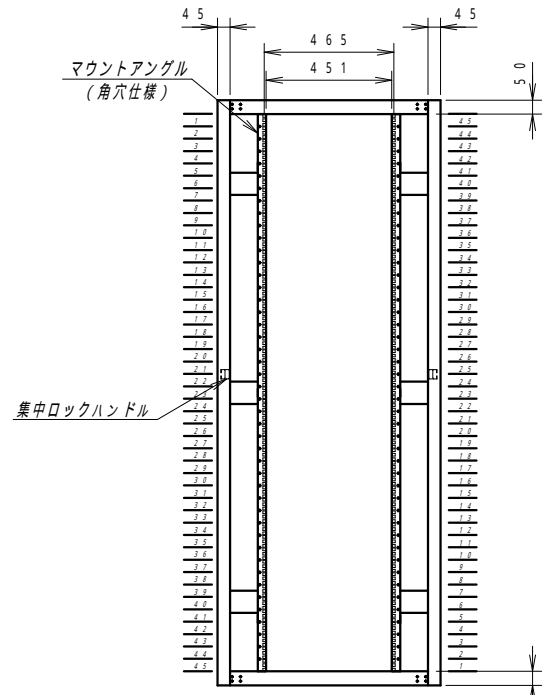
正面内観図
