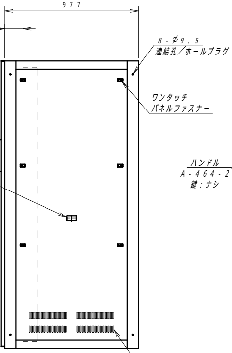
側面図
