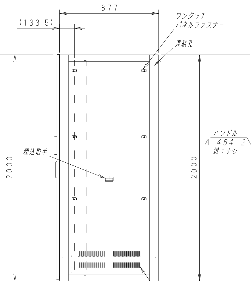
側面図
