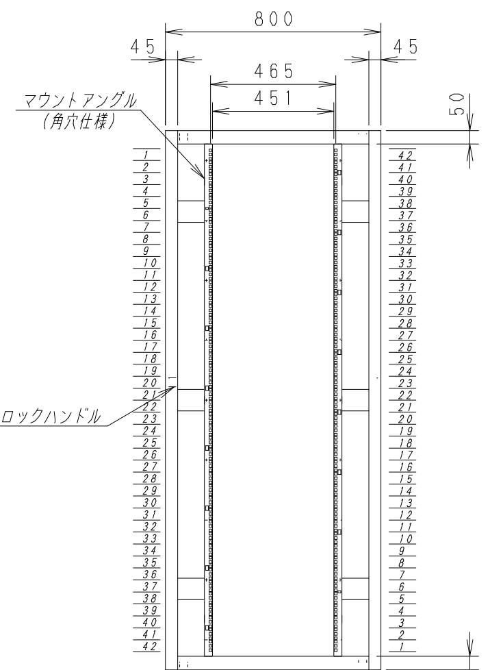
正面内観図
