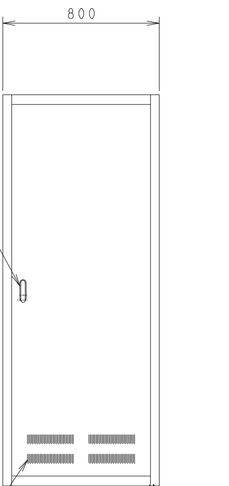
背面図
