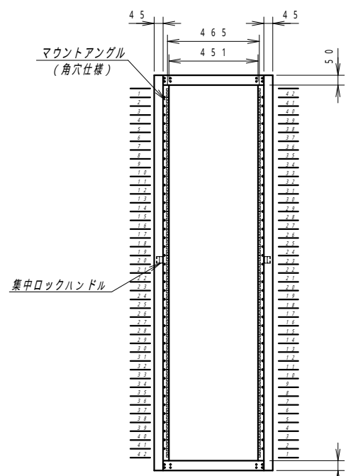
正面内観図
