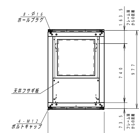
平面図
