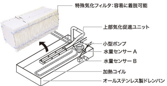
高性能ドレン酸化処理ユニット
