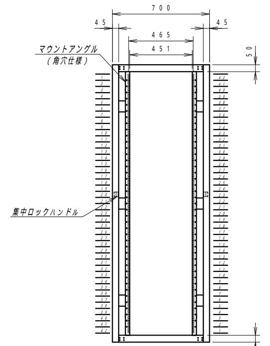
正面内観図
