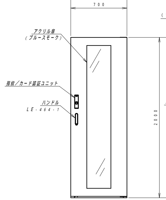
正面図
