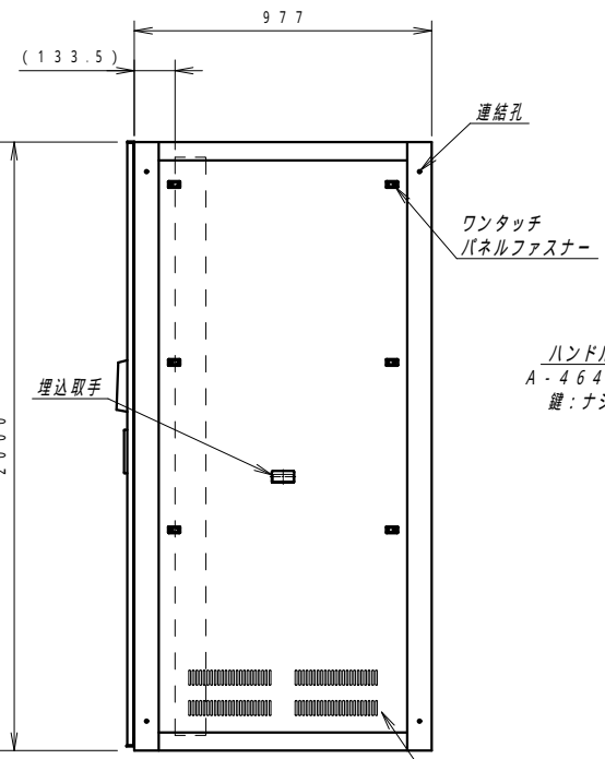
側面図
