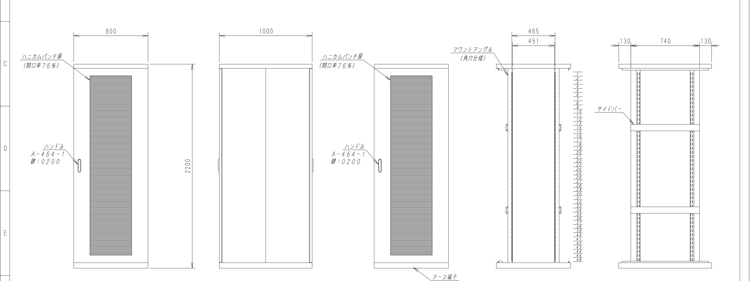
正面図 側面図 背面図 正面内観図 側面内観図
